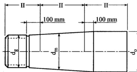
Pintle
