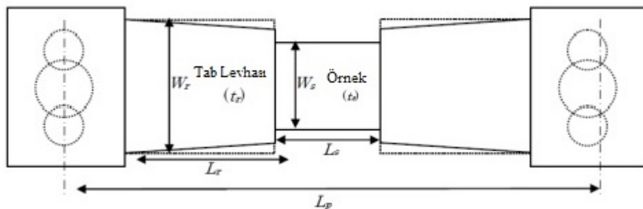
Şekil 1 Test numunesinin kavramsal görünüşü, tab ve yüklemeye jigi
