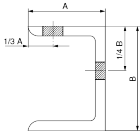
Şekil 3.5 Profiller
