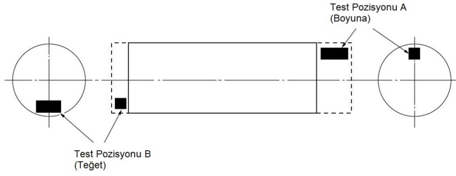
Şekil 5.1 Düz şaft
