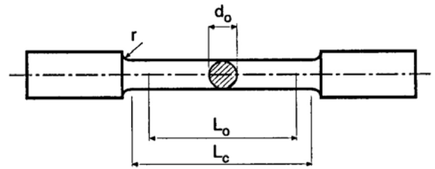
Şekil 2.1 Dairesel kesitli test numunesi
