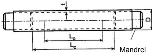
Şekil 2.3 Tam kesitli test numunesi
