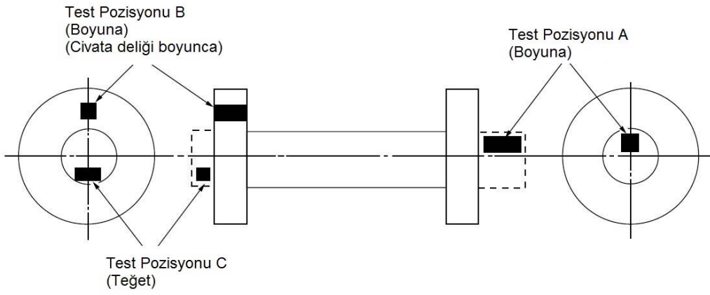
Şekil 5.2 Flençli şaft
