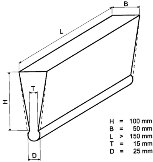
Şekil 11.1 Test parçası dökümü
