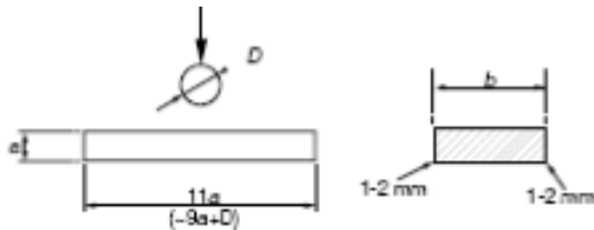
Şekil 2.7 Düz eğme test numunesi
