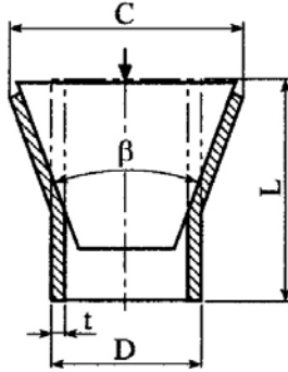
Şekil 2.10 Ağız genişletme testi
