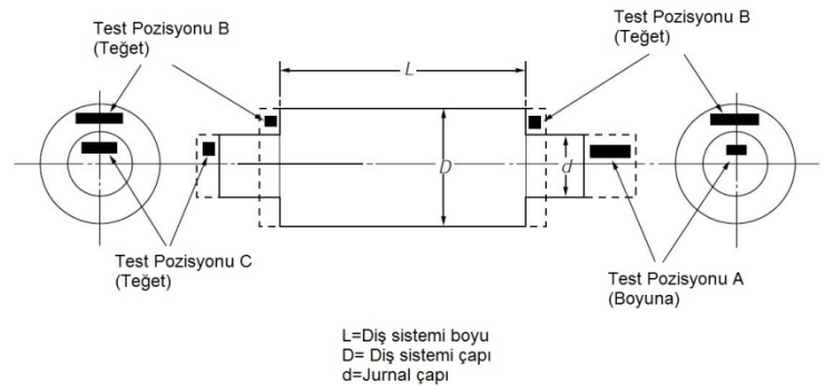
Şekil 5.5 Pinyon
