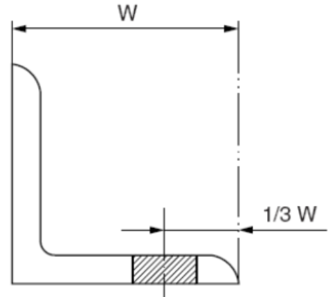
Şekil 3.4 Köşebentler
