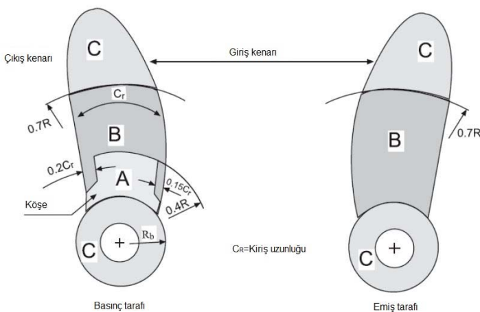
Şekil 11.3 Küçük kanat çalıklılığı olan birlikte dökülmüş pervanelerde tehlike oluşturacak bölgeler
