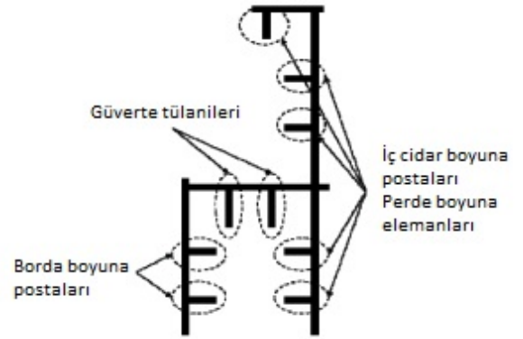
Şekil 3.14 Üst flenç boyuna yapısal elemanları
