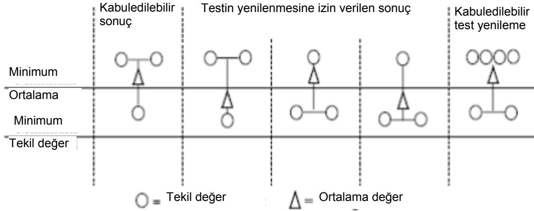
Şekil 3.12 Kabul/red ve testin yenilenme kriterleri diyagramı
