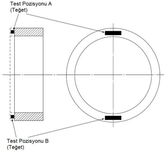
Şekil 5.7 Çark kasnakları
