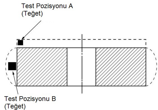
Şekil 5.6 Dişli çarklar
