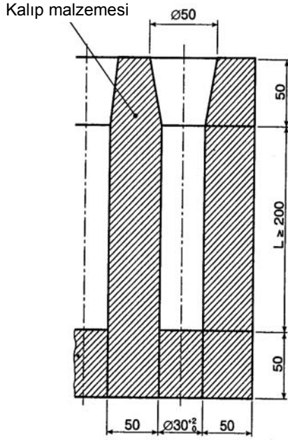
Şekil 7.4 Kır Dökme Demir için test parçası
