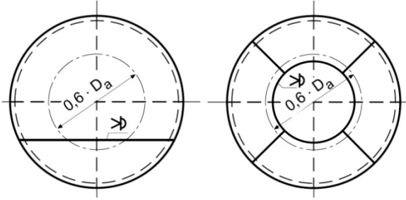
Şekil 12.10 Bombelik içindeki kaynak dikişi
