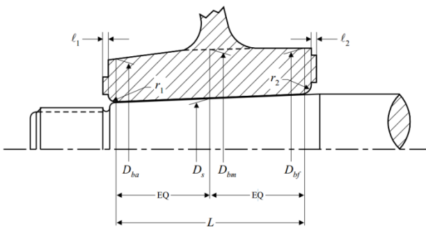
Şekil 8.3 Göbek ile şaft arasında teorik temas yüzeyi
