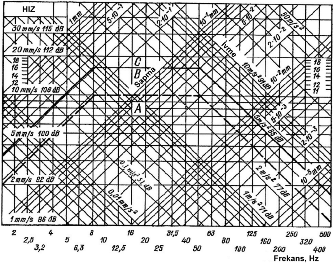
Şekil 1.7 Pistonlu kompresörler için titreşim standartları, - - - - A bölgesi üst sınırı, - - - - B bölgesi üst sınırı
