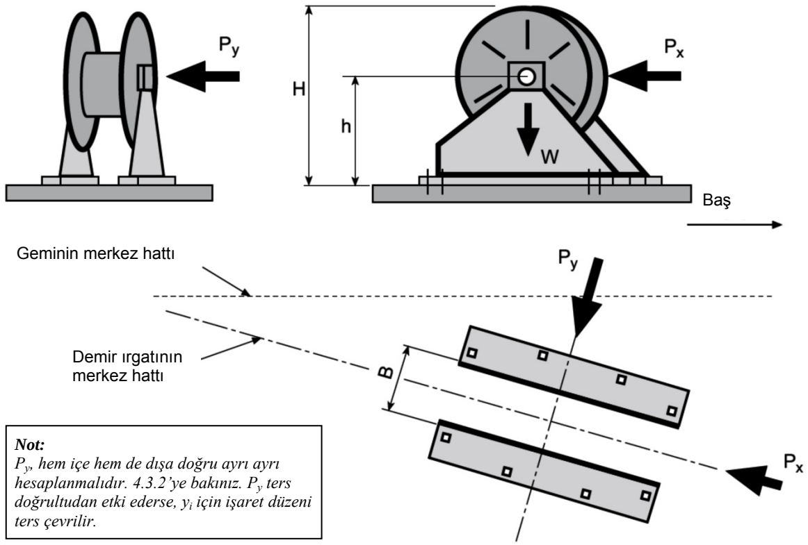
Şekil 11.1 Demir ırgatı yükleri
