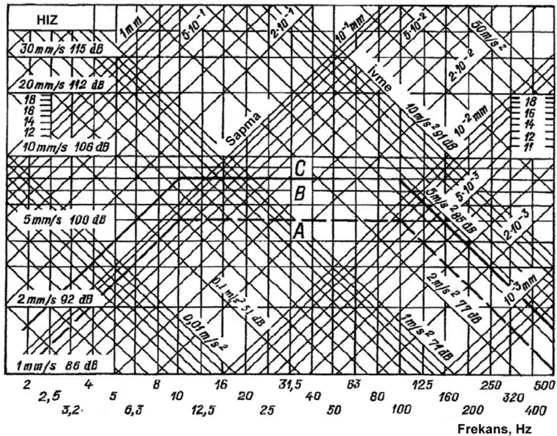
Şekil 1.5 Merkezkaç ayırıştırıcılar için titreşim standartları - - - - A bölgesi üst sınırı, ----- B bölgesi üst sınırı
