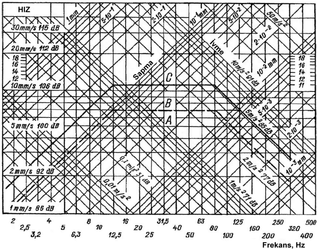
Şekil 1.3 Gücü 1.000 kW veya üzeri olan dizel jeneratörler ve şaft jeneratörleri için titreşim standartları - - - A bölgesi üst sınırı, ----- B bölgesi üst sınırı
