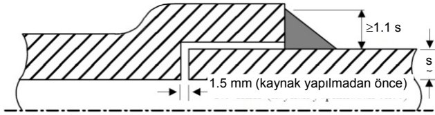
Şekil 16.2 Tipik manşon kaynağı
