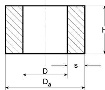
Şekil 9.1 Göbek boyutları
