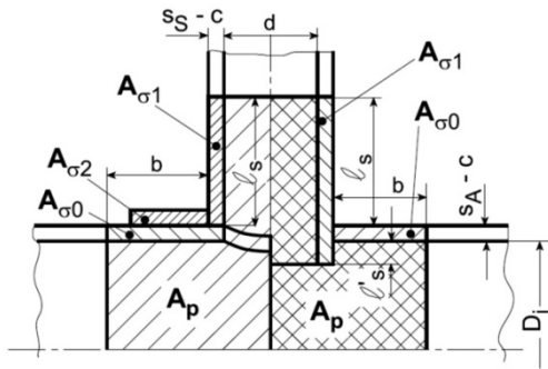
Şekil 12.2 Silindirik kabuktaki açıklık
