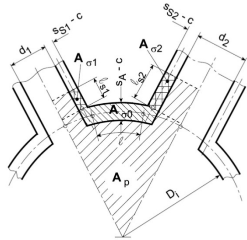
Şekil 12.9 Açıklıklardaki karşılıklı etkileşim
