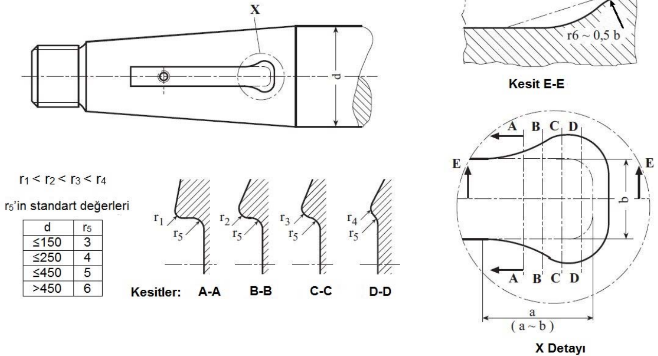
Şekil 5.1 Pervane şaftındaki kama yuvasının dizaynı
