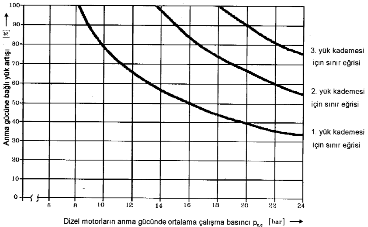
Şekil 2.16 4 stroklu dizel makinalarının, ortalama çalışma basıncının fonksiyonu olarak sıfır yükten nominal gücüne kadar kademe, kademe yüklenmesi için sınır eğrileri
