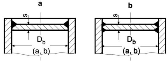
Şekil 12.14 Dairesel kaynaklı aynalar
