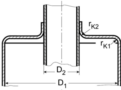
Şekil 12.21 Ortadan payandalı düz halka şeklindeki levhalar
