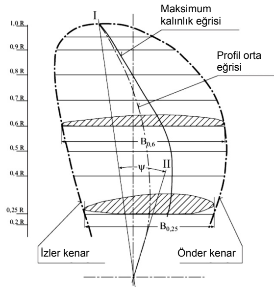
Şekil 8. 1 Kanat kesitleri ve maksimum çalıklık açısı
