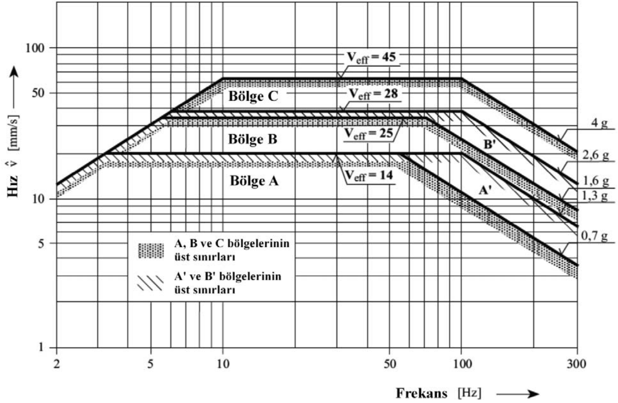
Şekil 1.1 Titreşim yüklerinin belirlenmesi için bölgeler
