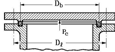
Şekil 12.13 Sızdırmazlık ringli dairesel levhalar
