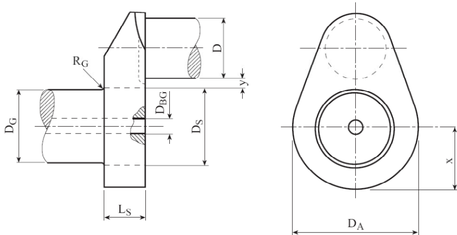
Şekil 2.12 Yarı-imalat krankşaft için krank dilimi
