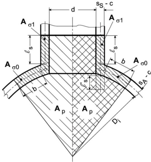
Şekil 12.8 Bombeli aynadaki açıklıklar
