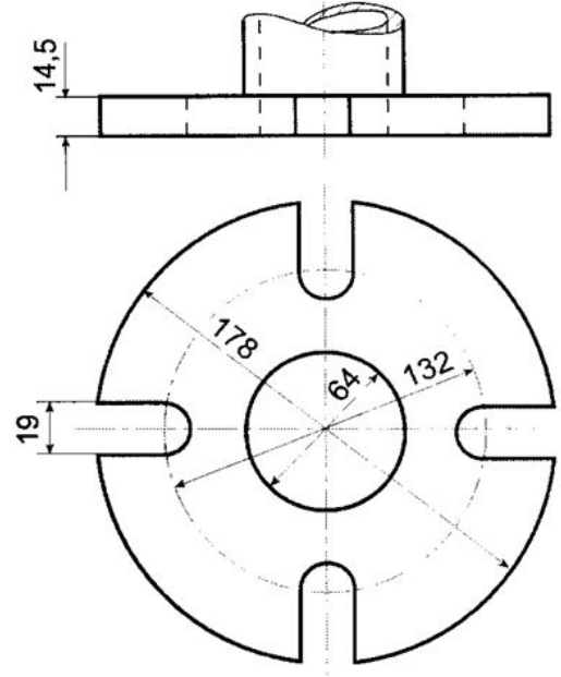
Şekil 18.1 Uluslararası yangın söndürme sahil bağlantısı
