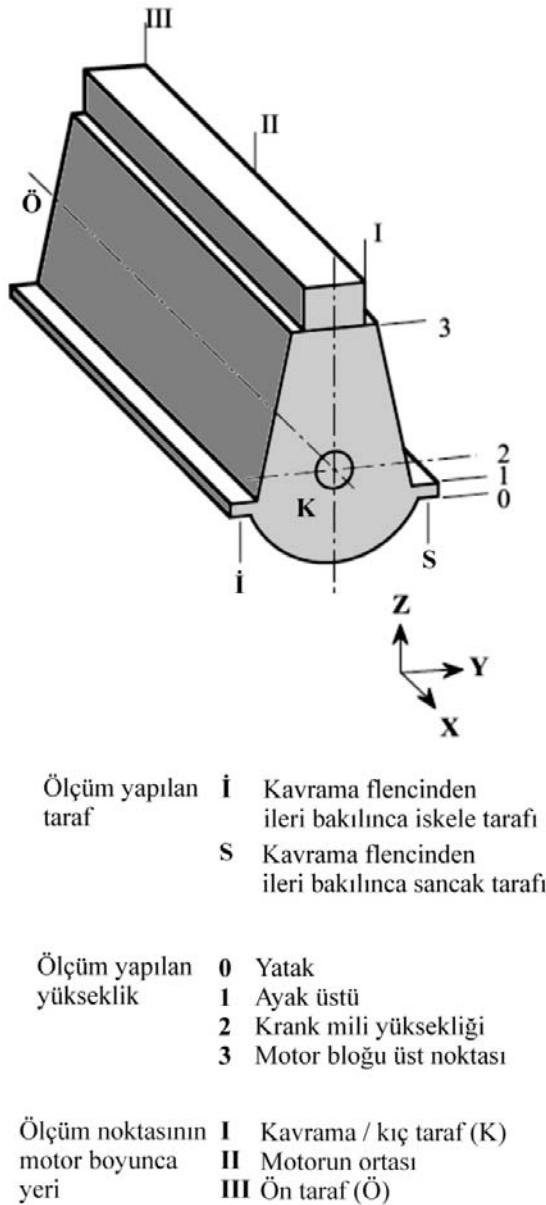
Şekil 1.8 Sıralı pistonlu motorların şematik görünüşü
