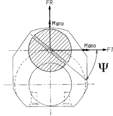
Şekil 2.5 Yağ deliği boyunca krankpin kesiti
