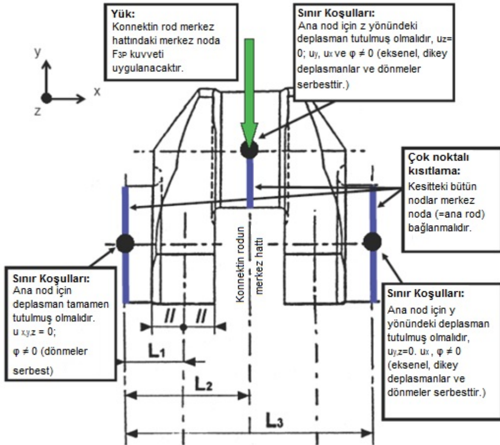
Şekil 2.10 Sıralı silindirli makinaların 3 noktalı eğilme yükleme durumu için sınır ve yükleme koşulları
