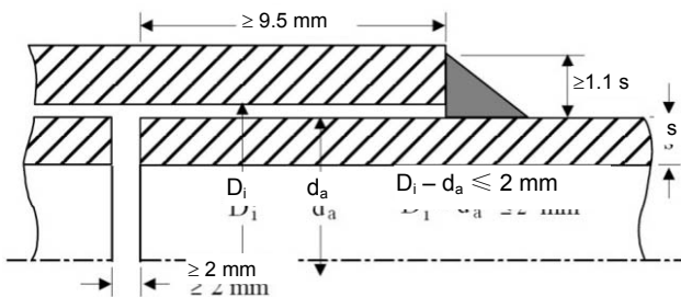
Şekil 16.3 Tipik kayıcı geçme bilezikli kaynaklı bağlantı
