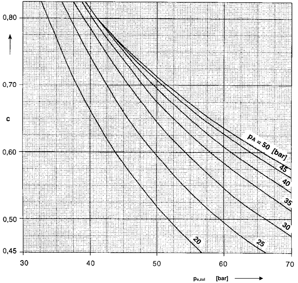
Şekil 2.17 Basınç düşürücü valfin bulunması durumunda (c) değeri
