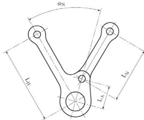
Fig. 2.2 Mafsallı tip biyel kolu
