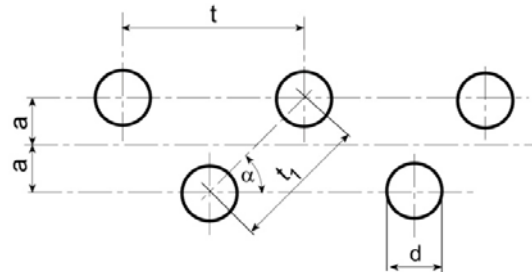
Şekil 12.25 Çapraz delikler için aralıklar
