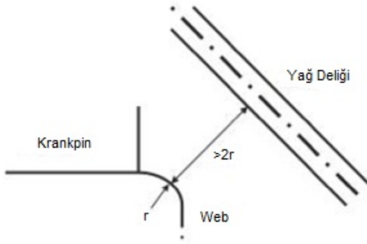
Şekil 2.7 Dolguya yakın yağ deliği
