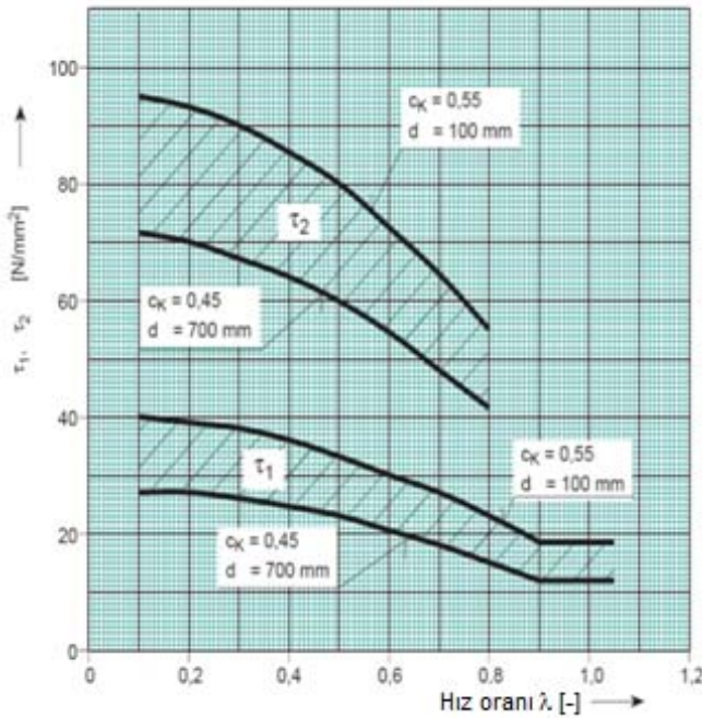
Şekil 6.2 Pervane şaftları için müsaade edilen burulma titreşim gerilmeleri
