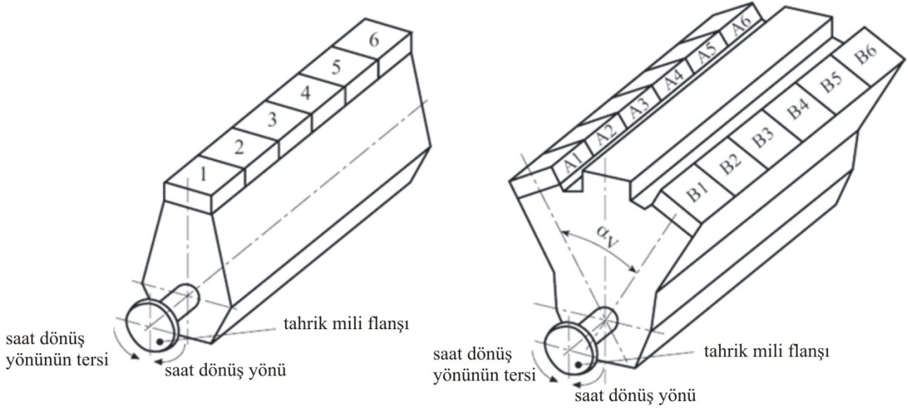
Fig. 2.1 Silindirlerin işaretlenmesi
