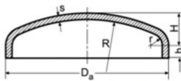
Delinmemiş bombeli aynalar
