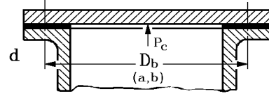
Şekil 12.12 Düz contalı dairesel levhalar
