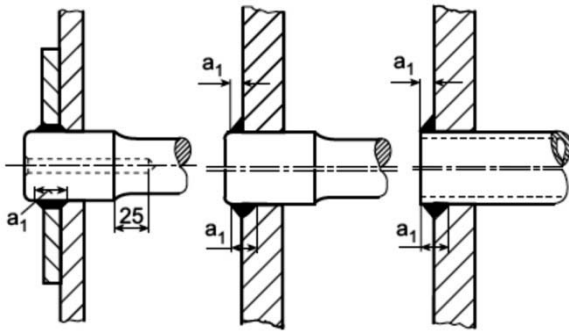
Şekil 12.22 Şekil 12.23 Şekil 12.24 Payandalar, payanda boruları ve payanda civatalarının kaynak parametreleri
