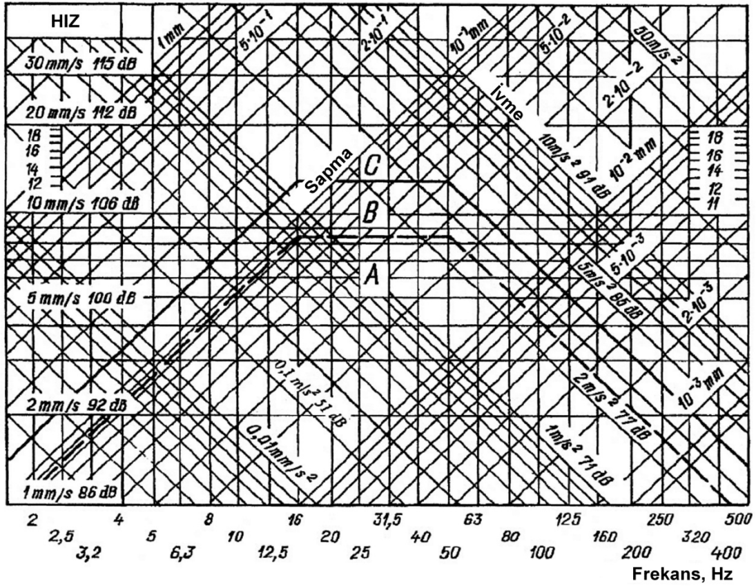
Şekil 1.6 Fanlar için titreşim standartları - - - - A bölgesi üst sınırı, - - - - B bölgesi üst sınırı
