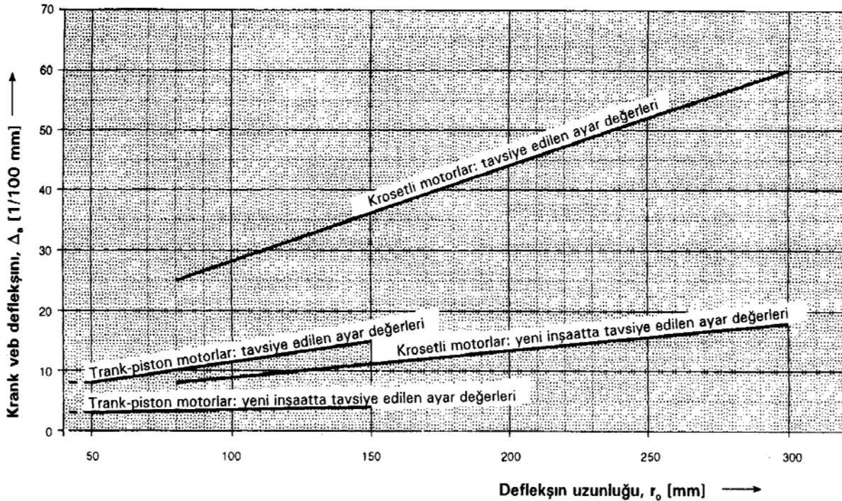
Şekil. 2.18 Krank veb sapması için başvuru değerleri
