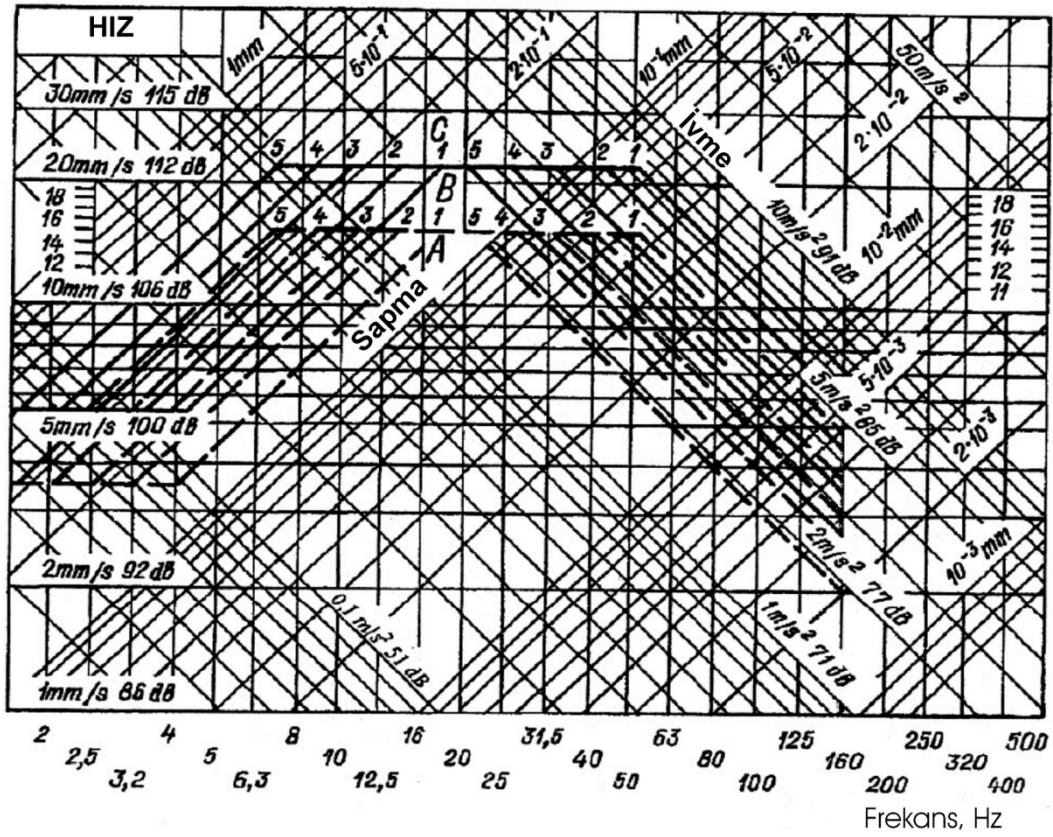
Şekil 1.2 İçten yanmalı makinalar için titreşim standartları (strok boyu 1- 30 cm'den az, 2- 30~70 cm arası, 3- 71~140 cm arası, 4- 141~240 cm arası, 5- 240 cm'den büyük) - - - A bölgesi üst sınırı, ----- B bölgesi üst sınırı
