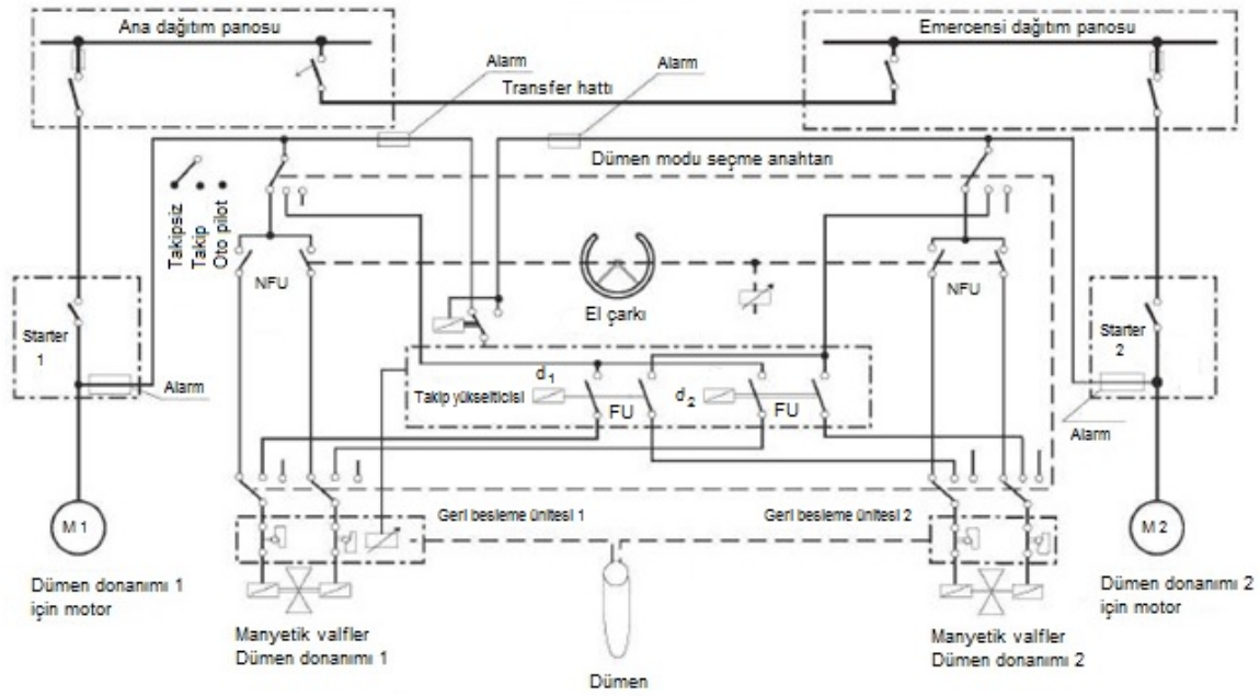
Şekil 9.4 Çift olmayan takip kontrol ve oto pilot sistemi prensip şeması, takip kontrol oto pilotta veya diğer ek kontrolde.
