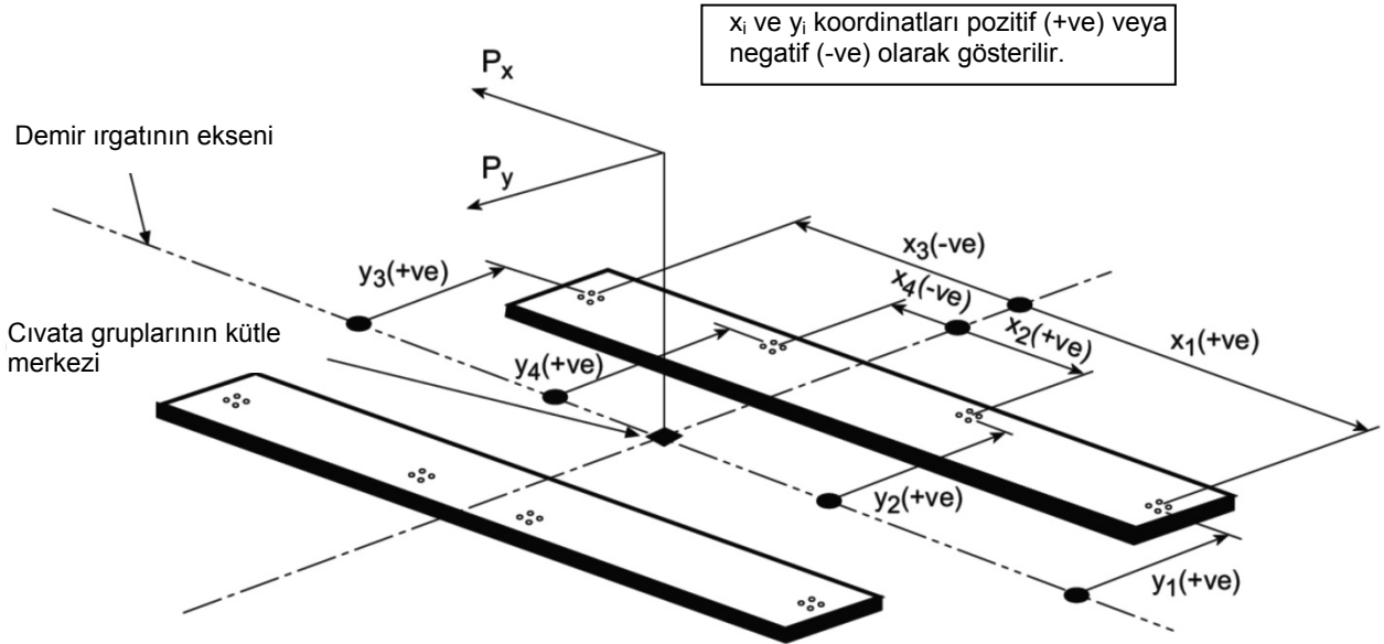
Şekil 11.2 Kuvvetlerin ve ağırlıkların doğrultusu ve işaret düzeni
