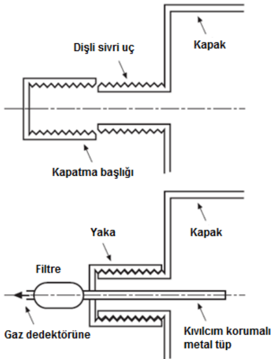
Şekil 12.2 Gaz örnek alma noktaları
