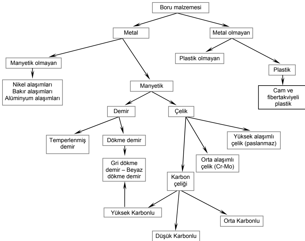
Şekil 16.1 Boruların üretildikleri malzeme türleri
