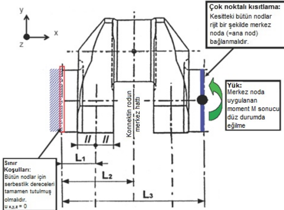
Şekil 2.9 Saf eğilme yükleme durumu için sınır ve yükleme koşulları
