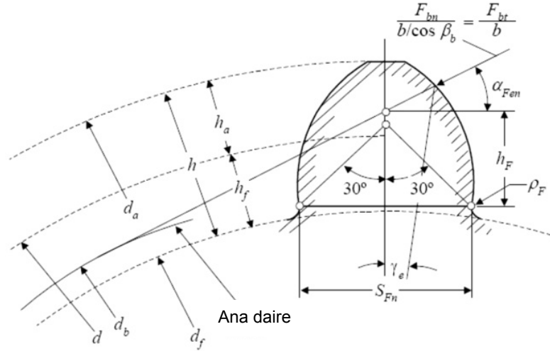
Şekil 7.1 Tipik bir dış silindirik dişlisinin diş profilinin en kesiti üzerindeki ölçümler
