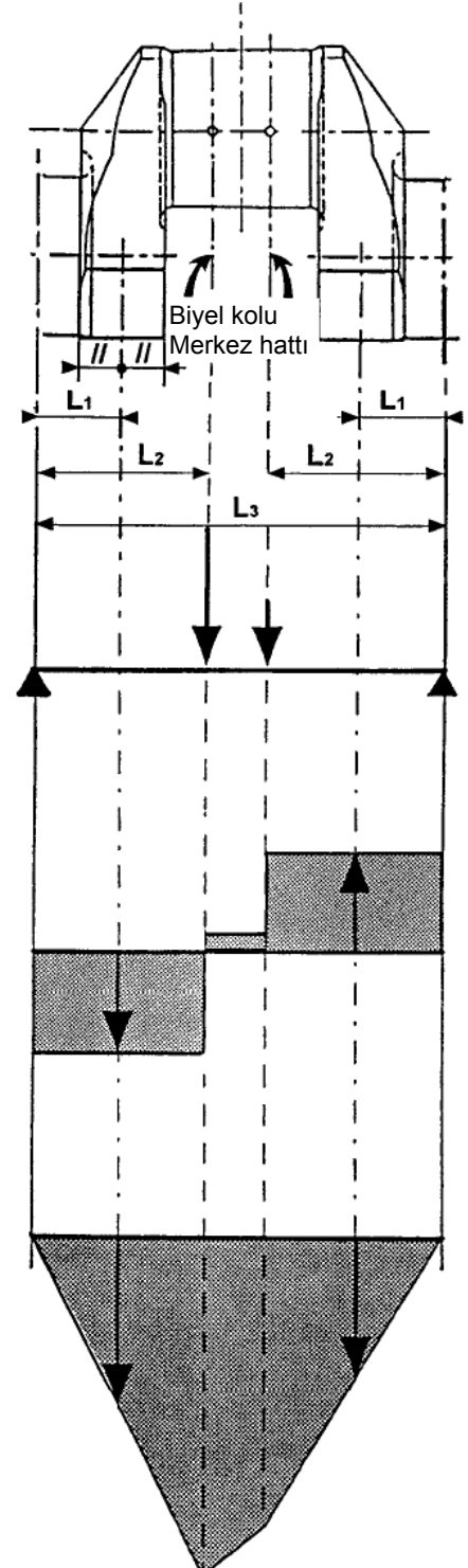
Şekil. 2.4 V-tipi iki bitişik biyel kollu makina için krank dilimi
