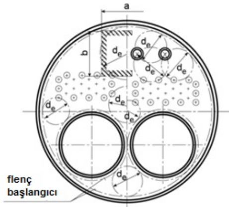
Şekil 12.20 Takviyeli düz levhalar
