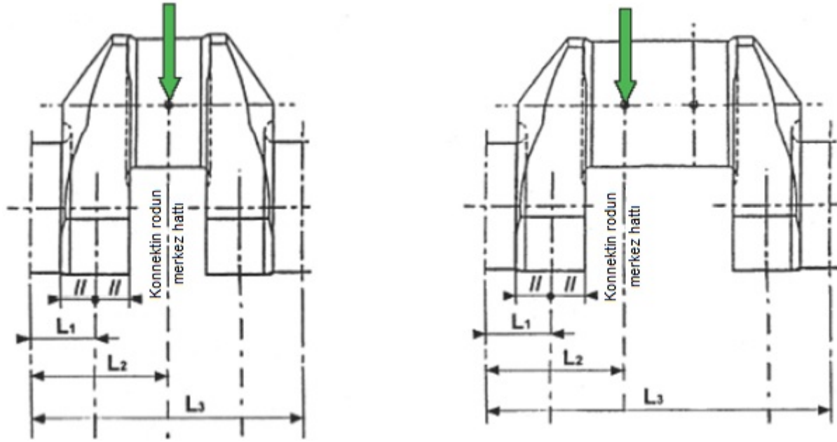
Şekil 2.11 Sıralı silindirli ve V tipi makinalarda yükleme uygulamaları
