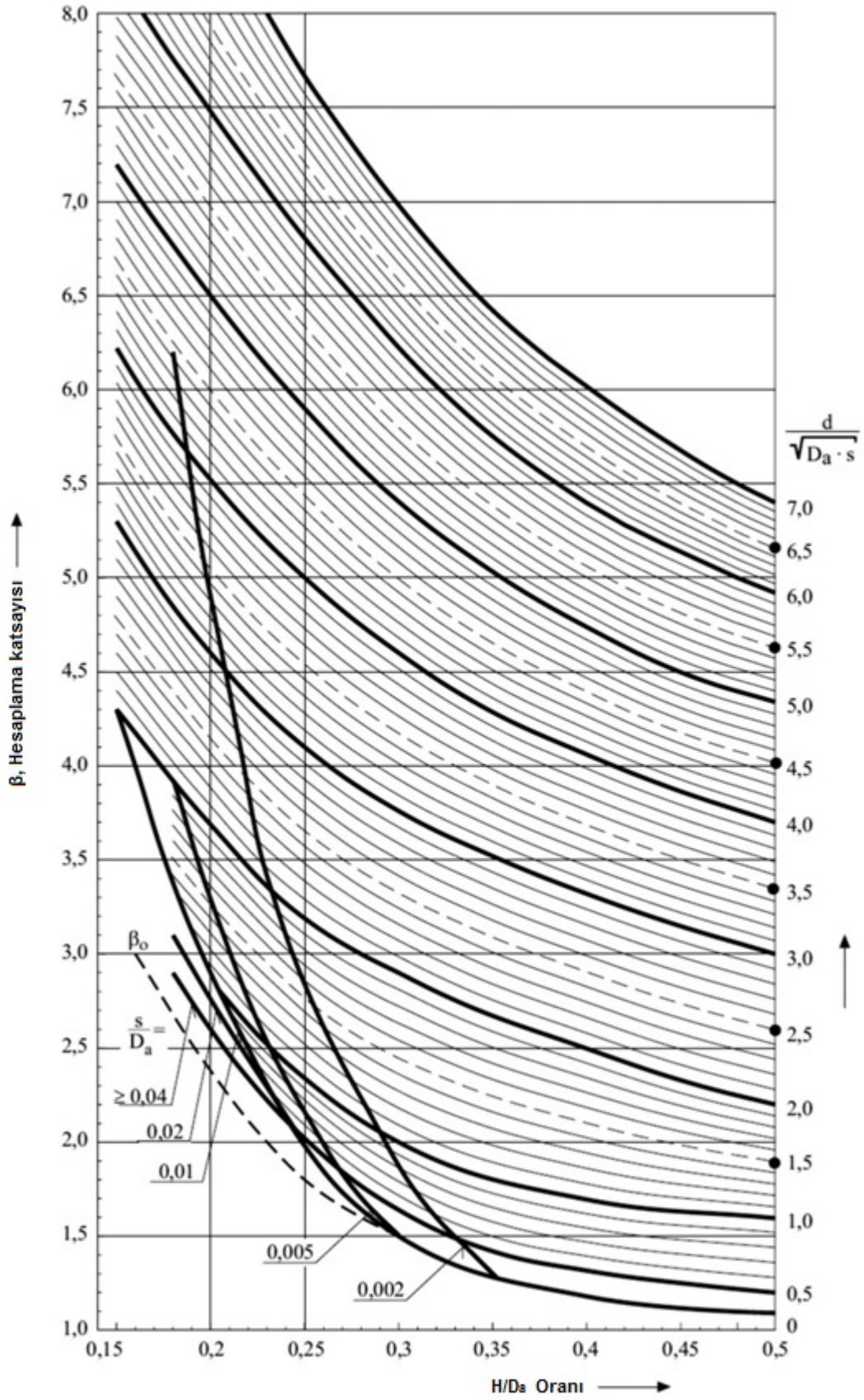
Şekil 12.7 Bombeli aynaların tasarımı için \beta katsayıları
