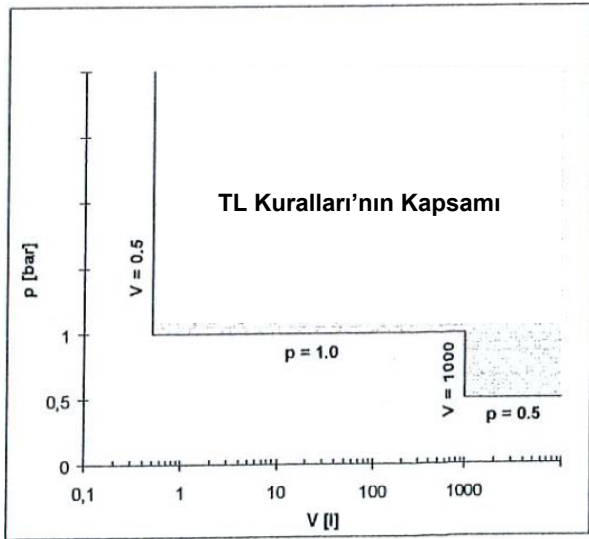
Şekil 14.1 Basınçlı kaplar ve ısı değiştiriciler için TL Kuralları'nın kapsamı
