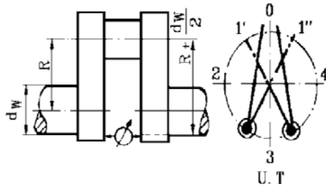
Şekil. 2.19 Krank veb sapması ölçüleri
