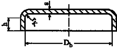
Şekil 12.11 Düz, dairesel ve flençli aynalar
