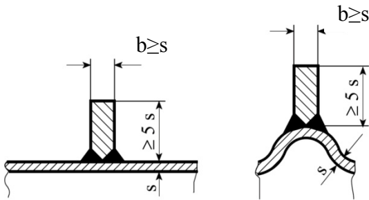
Şekil 12.4 Etkin takviyeler
