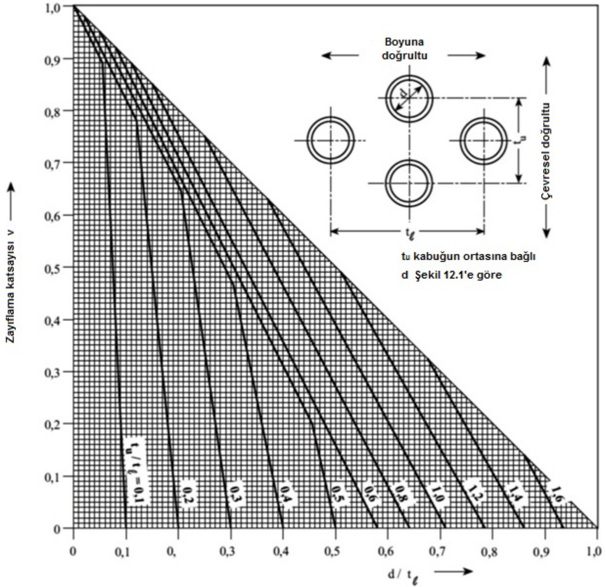
Şekil 12.27 Simetrik olarak şaşırtılmış delik sıralı silindirik kabuklar için zayıflama katsayısı v
