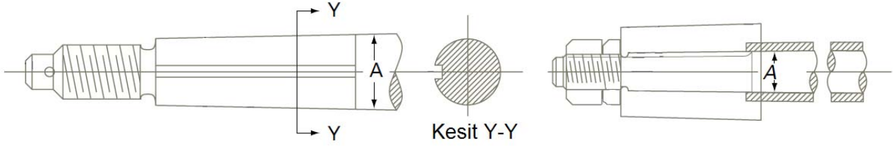
Şekil 5.2 Pervane şaft nihayetinin tipik detayı
