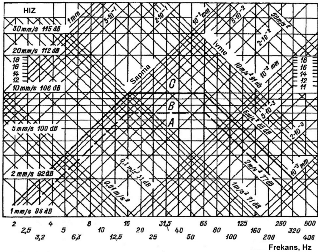
Şekil 1.4 Pompalar için titreşim standartları - - - - A bölgesi üst sınırı, ----- B bölgesi üst sınırı
