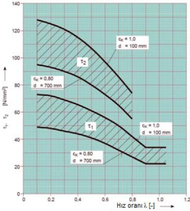
Şekil 6.1 Ara şaftlar için müsaade edilen burulma titreşim gerilmeleri
