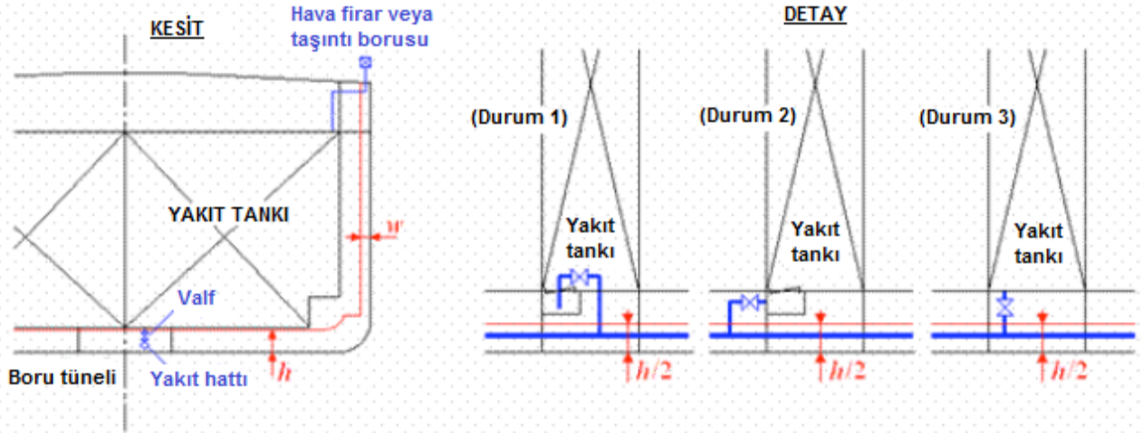
Şekil 16.5 Yakıt tankları için hava firar boruları, taşıntı boruları ve valfler
