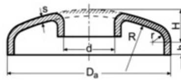
Menhollü bombeli aynalar
