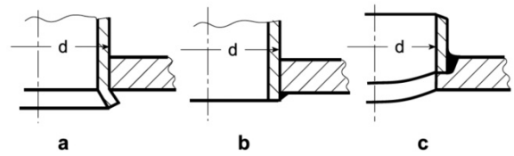
Şekil 12.1 Delik çapı ve boru iç çapı
