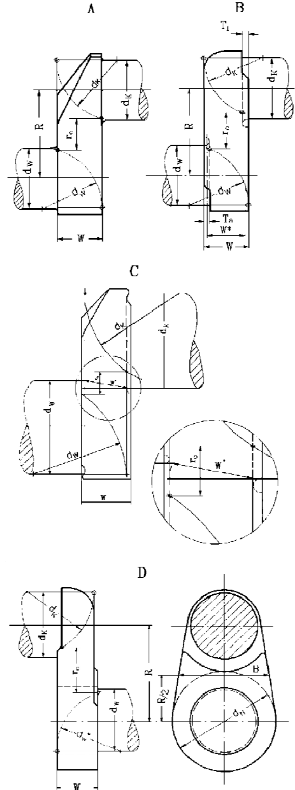
Şekil 2.20 Dövülmüş (A, B ve C) ve yarı-imalat (D) krankshaft tipleri
