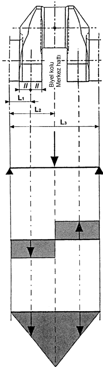
Şekil. 2.3 Sıralı tipte makina için krank dilimi
