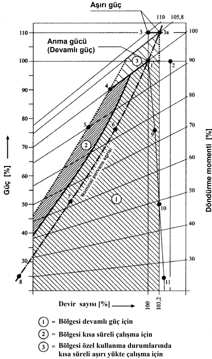
Şekil 2.15 Güç / Devir sayısı diyagramı
