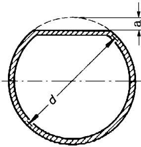
Şekil 12.5 Ovallık parametreleri
