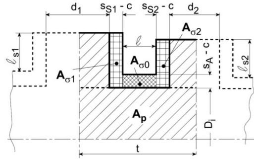
Şekil 12.3 Açıklıklardaki karşılıklı etkileşim
