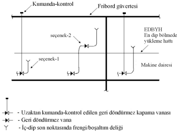
Şekil 16.4 SOLAS'a göre fribord güvertesinin altındaki mahallerden bordadan dışarı boşaltım ve vana yerleşimleri
