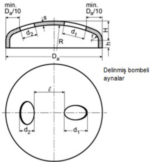
Şekil 12.6 Payandasız bombeli aynalar için parametreler
