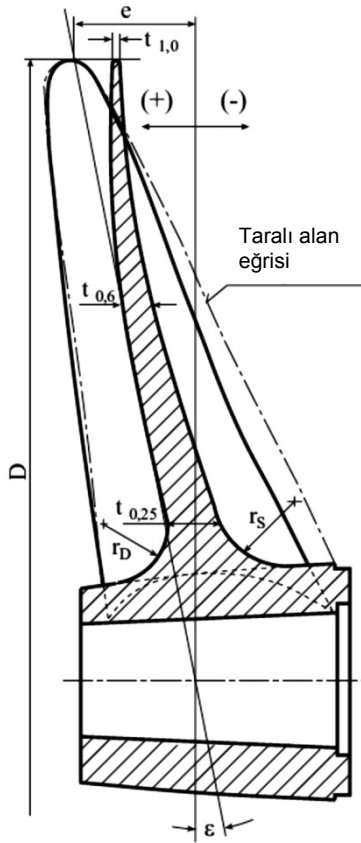
Şekil 8. 2 Eğiklik ve eğiklik açısı
